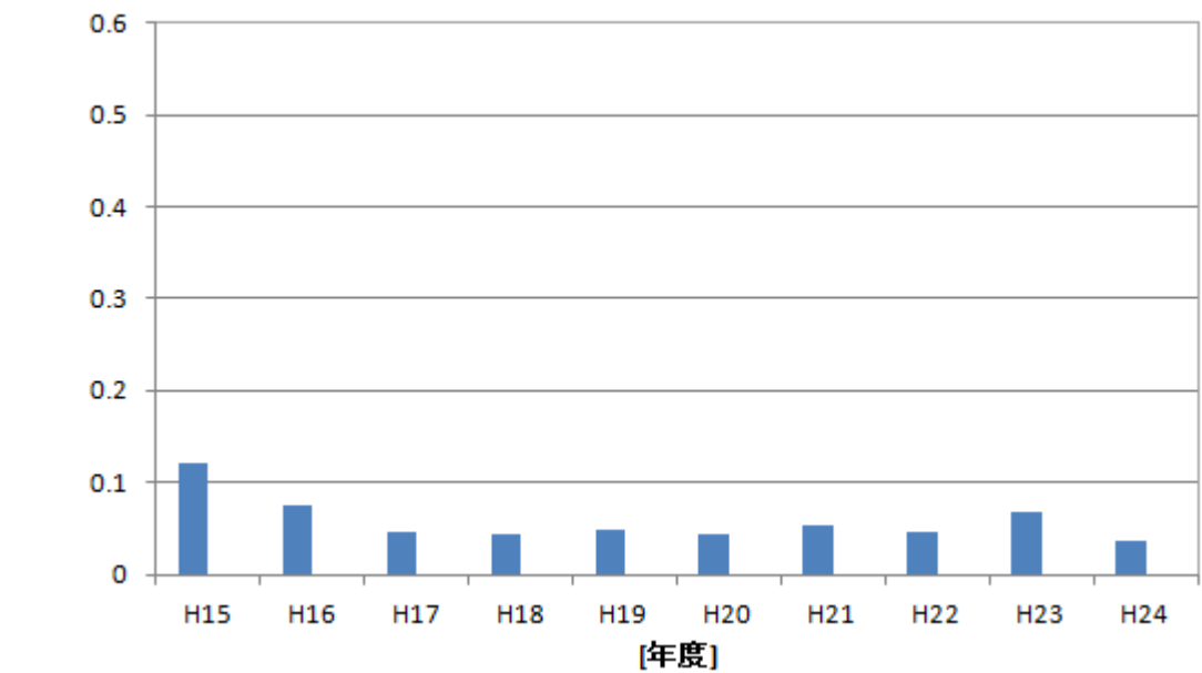
■大気中のダイオキシン類濃度の経年変化 [pg-TEQ/m³]
